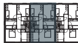
VERDIEPINGSPLAN
